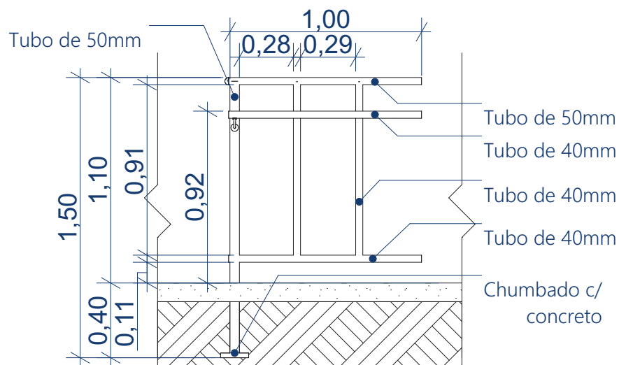
02 Módulo 1 c/ corrimão 1:20
