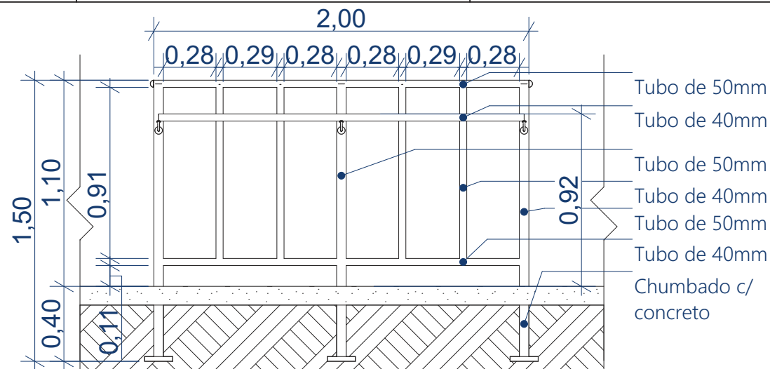
01 Guarda-corpo c/ corrimão 1:20
