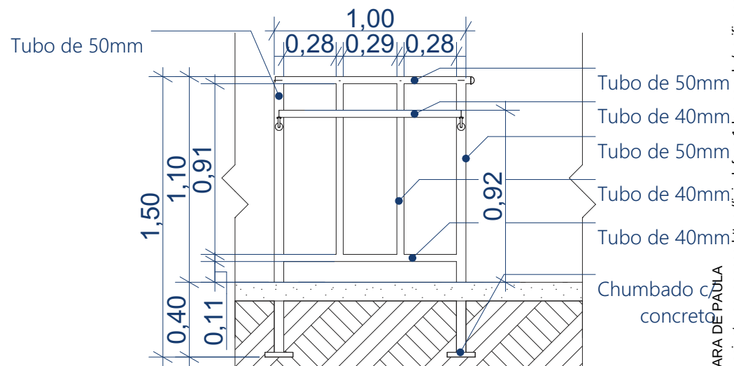
03 Módulo 2 c/ corrimão 1:20
